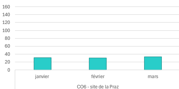
CO6 : Débits des eaux d'exhaure en entrée de STE (L/s)
