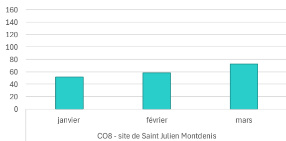
CO8 : Débits des eaux d'exhaure en entrée de STE (L/s)
