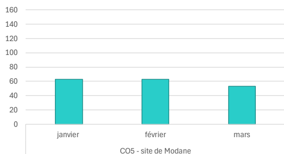
CO5 : Débits des eaux d'exhaure en entrée de STE (L/s)
